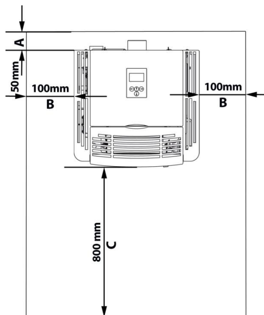
Illustration 2 : Distances de sécurité
