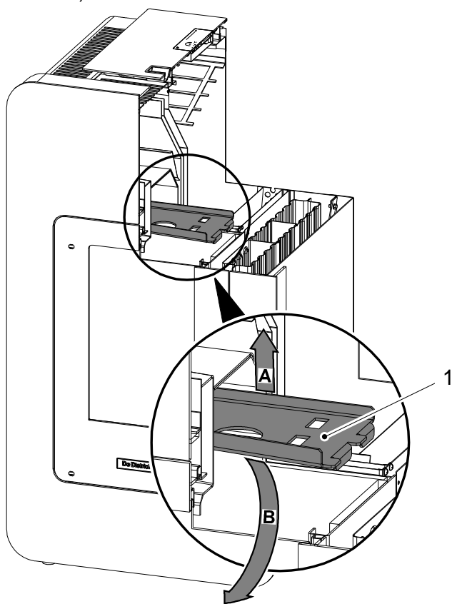
Illustration 8a : démontage de la plaque déflectrice
