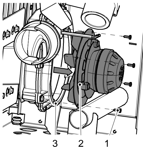
Illustration 9 : Ventilateur d'extraction des fumées
