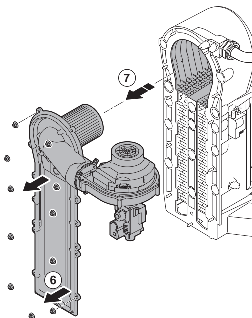
Fig.38 Dépose de la plaque avant, du ventilateur et du brûleur
