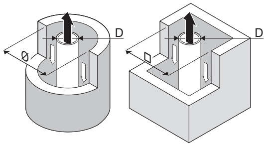
Fig.23 Dimensions minimales de la gaine ou du conduit C 93 , C 93X
