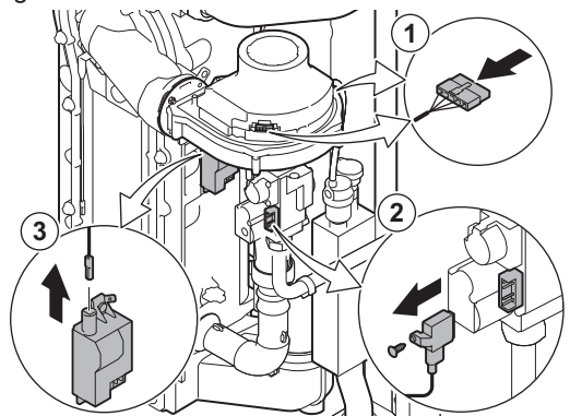
Fig.36 Débranchement du ventilateur
