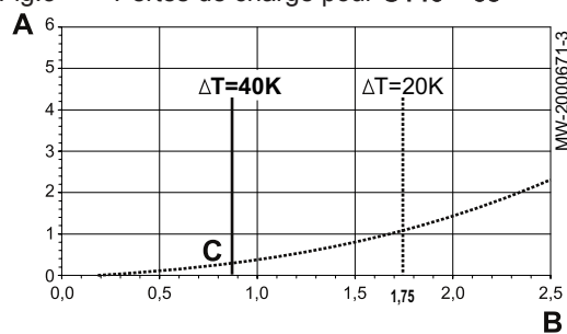
Fig.4 Pertes de charge pour C140 – 90
