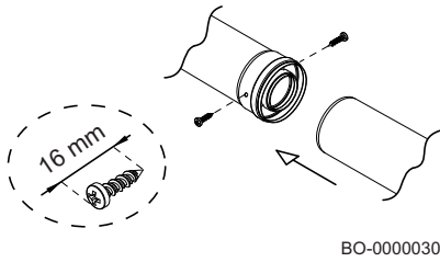
Fig.29 Fixation des conduits concentriques à l'aide de vis
