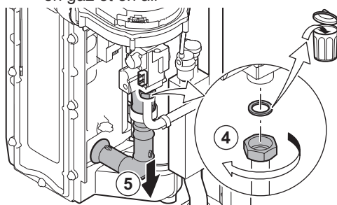
Fig.37 Retrait des conduites d'alimentation en gaz et en air
