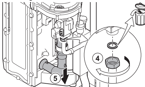
Fig.41 Retrait des conduites d'alimentation en gaz et en air
