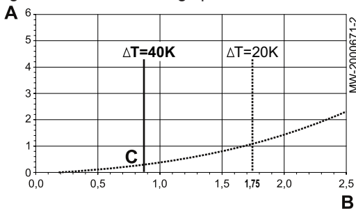
Fig.2 Pertes de charge pour C140 – 45
