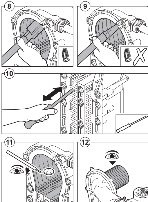
Fig.39 Nettoyage de l'échangeur de chaleur
