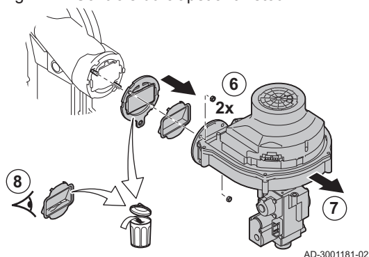
Fig.42 Contrôle du clapet anti-retour
