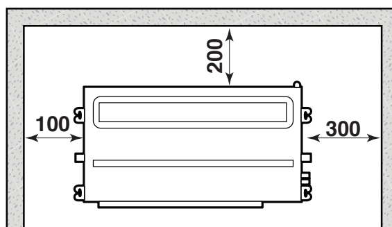
Vue de dessus (mm)
