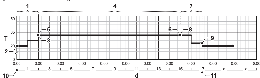
Fig.60 Courbe de séchage de la chape
