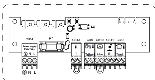
Fig.38 Raccordements de la carte de la chaudière
