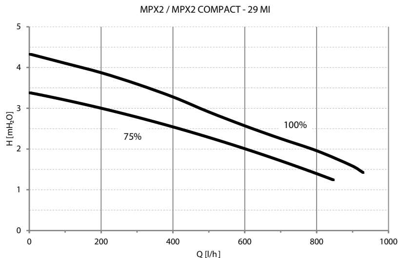
Fig.12 Graphique de la hauteur manométrique résiduelle de la pompe pour le modèle de chaudière 29 MI
