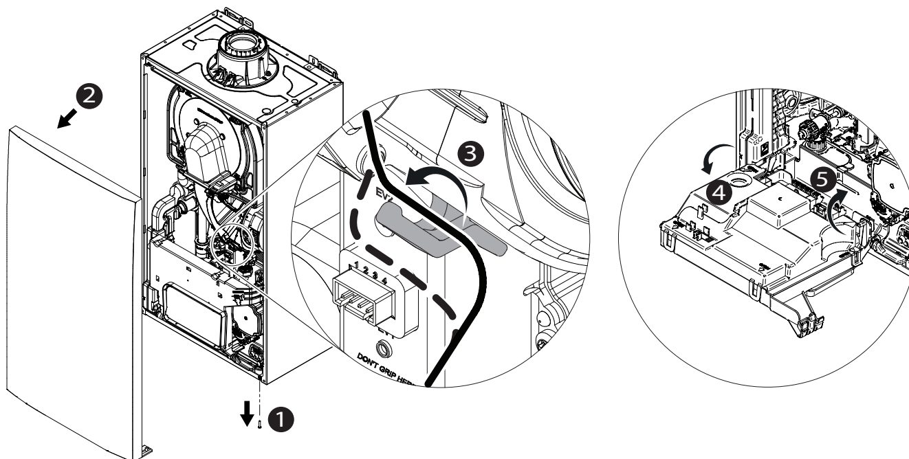
Fig.36 Accès aux raccordements électriques
