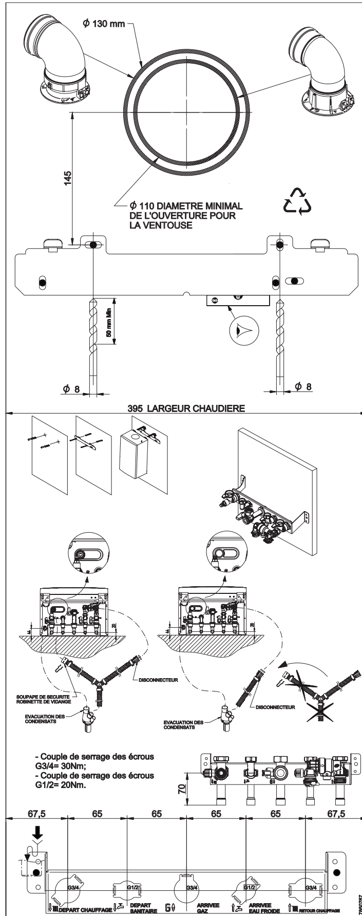
Fig.4 Gabarit sur papier modèle mixte Chauffage + Eau chaude sanitaire MPX2 COMPACT
