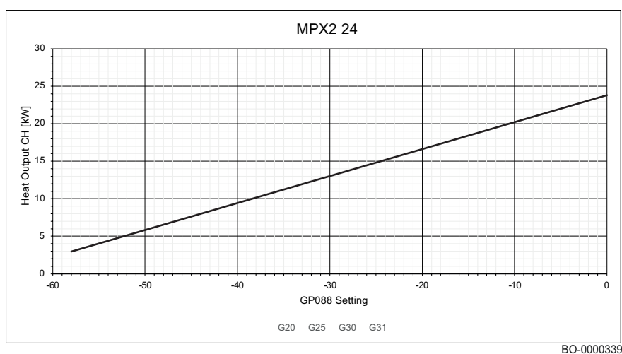
Fig.56 Graphique pour MPX2 - 24
