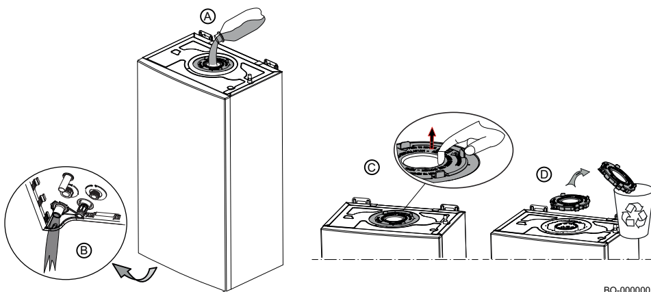
Fig.42 Méthode de remplissage du siphon avant l'installation du conduit
