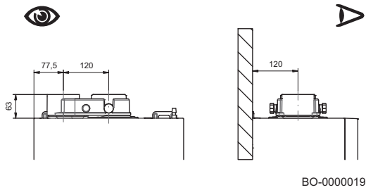
Fig.31 Type de conduits d'évacuation/ d'admission séparés
