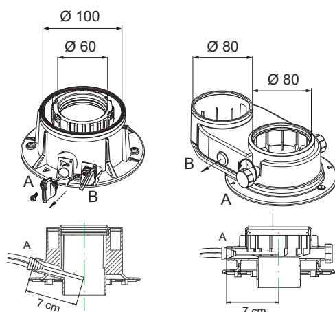
Fig.46 Type de raccords — point de mesure des gaz de combustion
