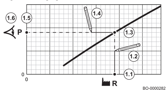
Fig.54 Réglage d'usine
