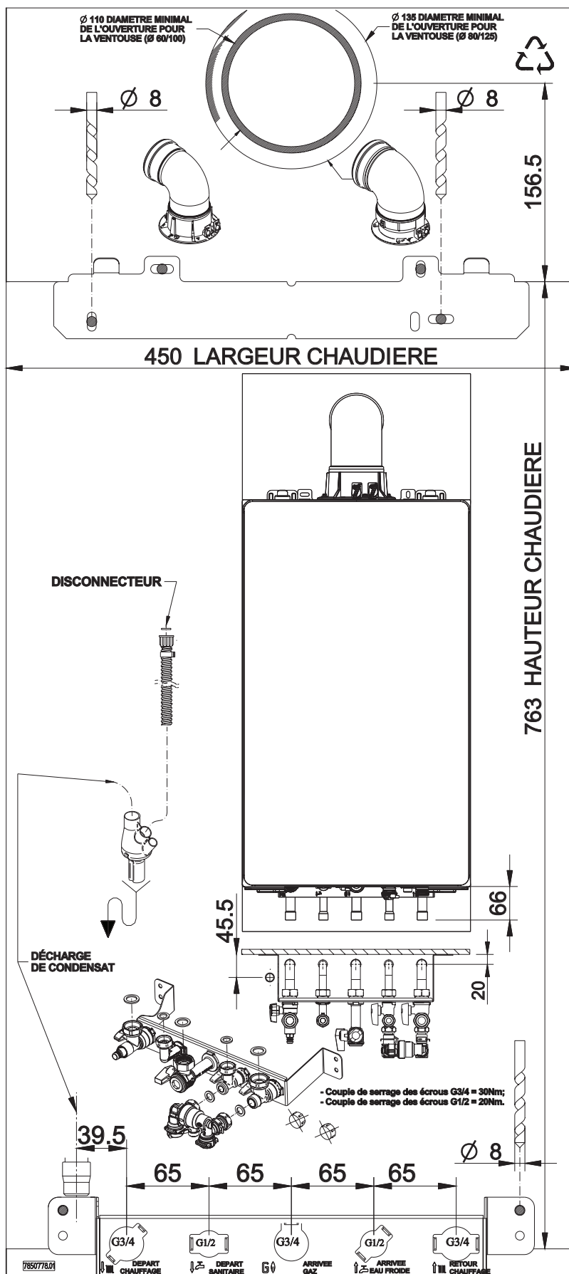
Fig.3 Gabarit sur papier modèle mixte Chauffage + Eau chaude sanitaire MPX2
