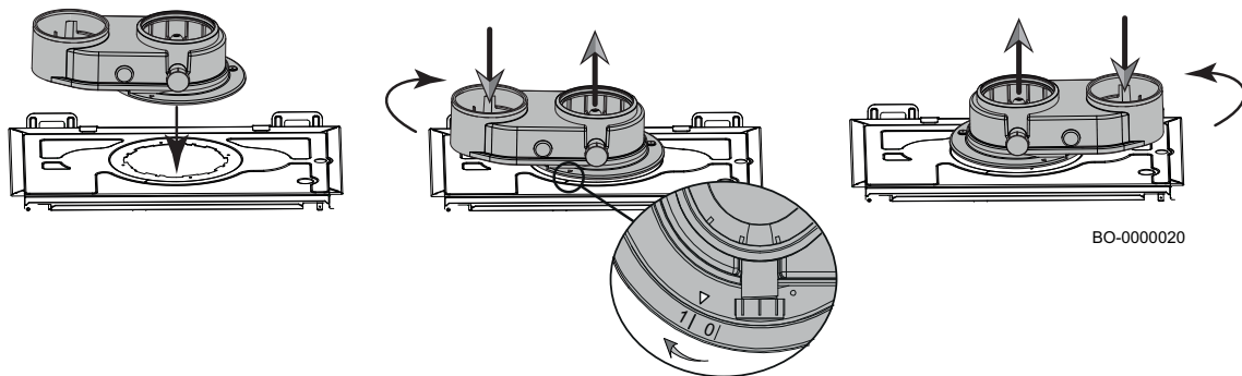
Fig.32 Installation des conduits séparés
