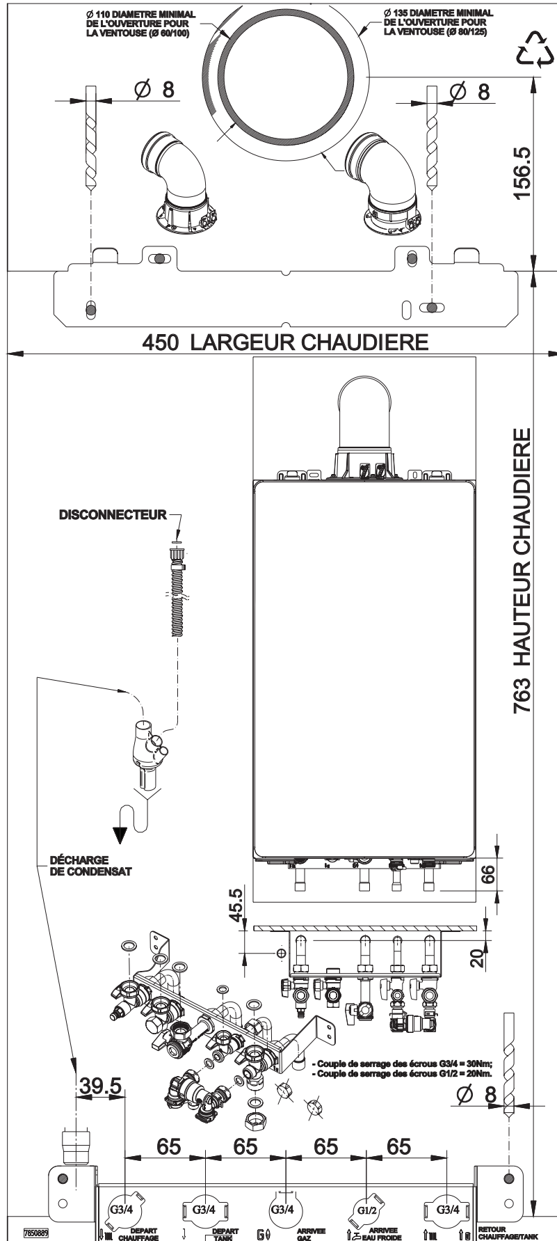
Fig.2 Gabarit sur papier du modèle Chauffage seulement MPX2
