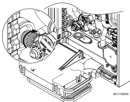
Fig.44 Vidanger l'installation
