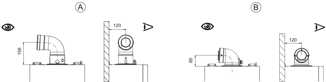
Fig.29 Type de conduits d'évacuation/d'admission concentrique
