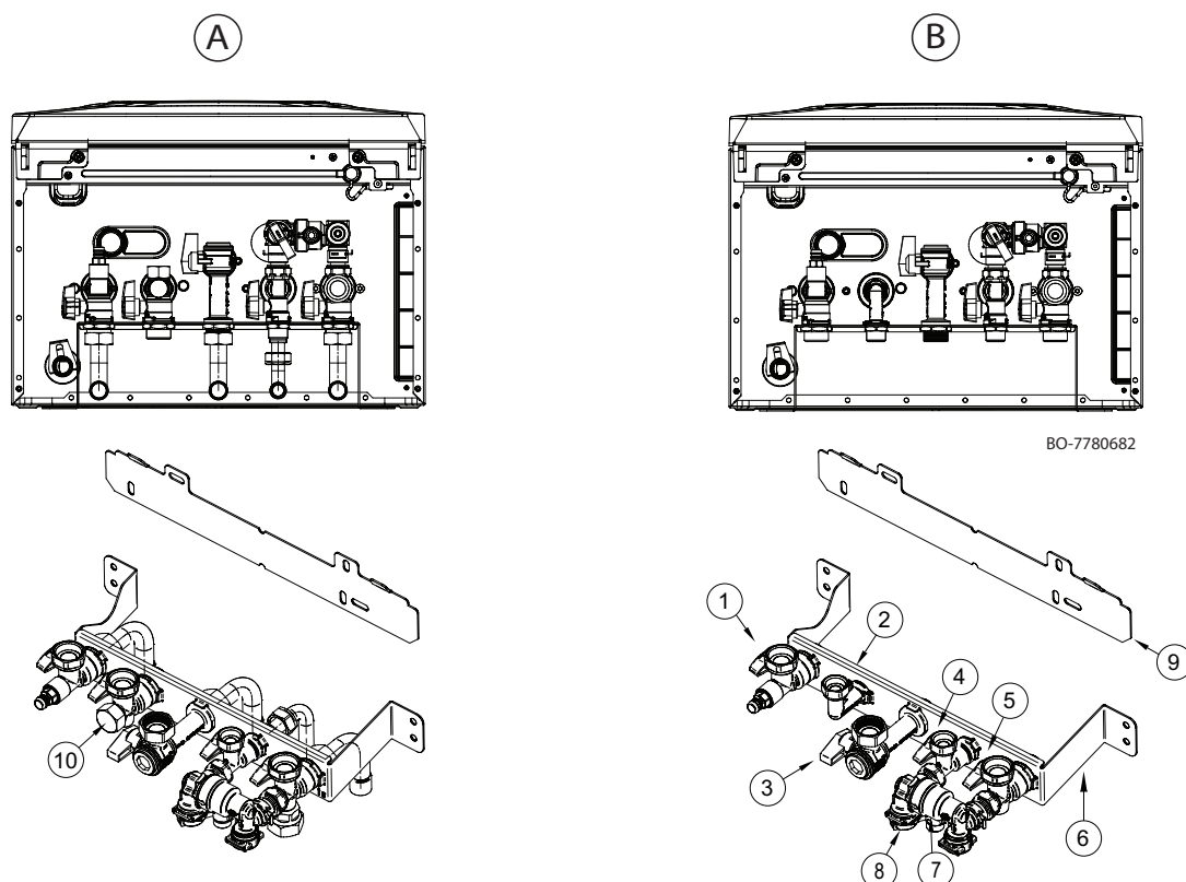
Fig.21 Description des composants sur la platine de raccordement
