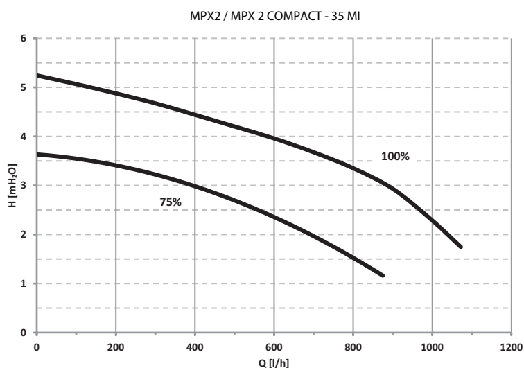
Fig.13 Graphique de la hauteur manométrique résiduelle de la pompe pour le modèle de chaudière 35 MI
