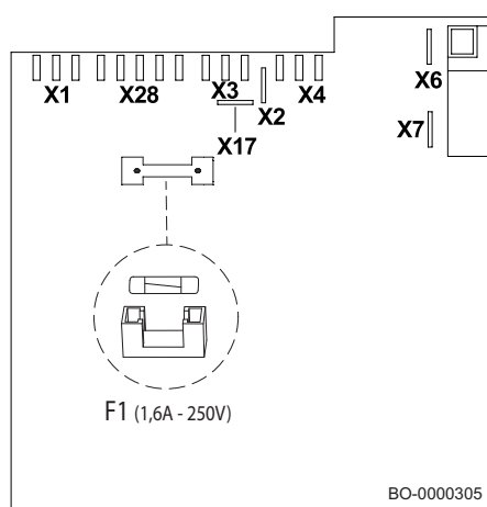
Fig.39 Emplacement du porte-fusible
