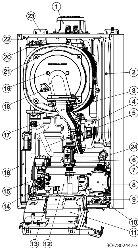
Fig.8 Chaudière en chauffage seul (pièce hydrobloc)
