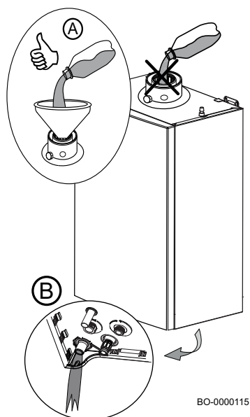
Fig.43 Méthode de remplissage du siphon avec le conduit installé
