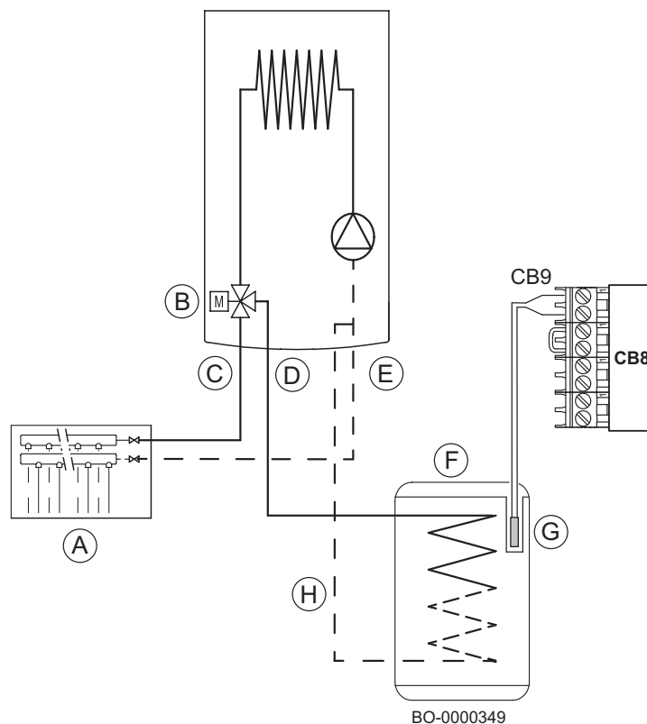
Fig.22 Raccordement du ballon d'ECS
