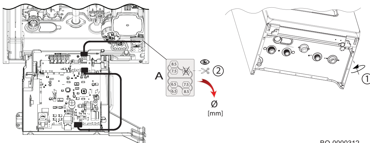
Fig.38 Raccordements de la carte de la chaudière
