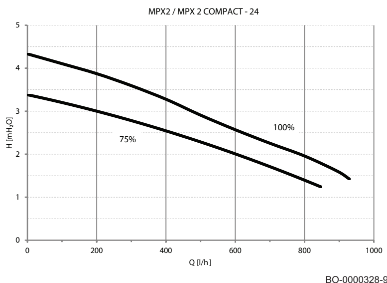
Fig.11 Graphique de la hauteur manométrique résiduelle de la pompe pour le modèle de chaudière 24
