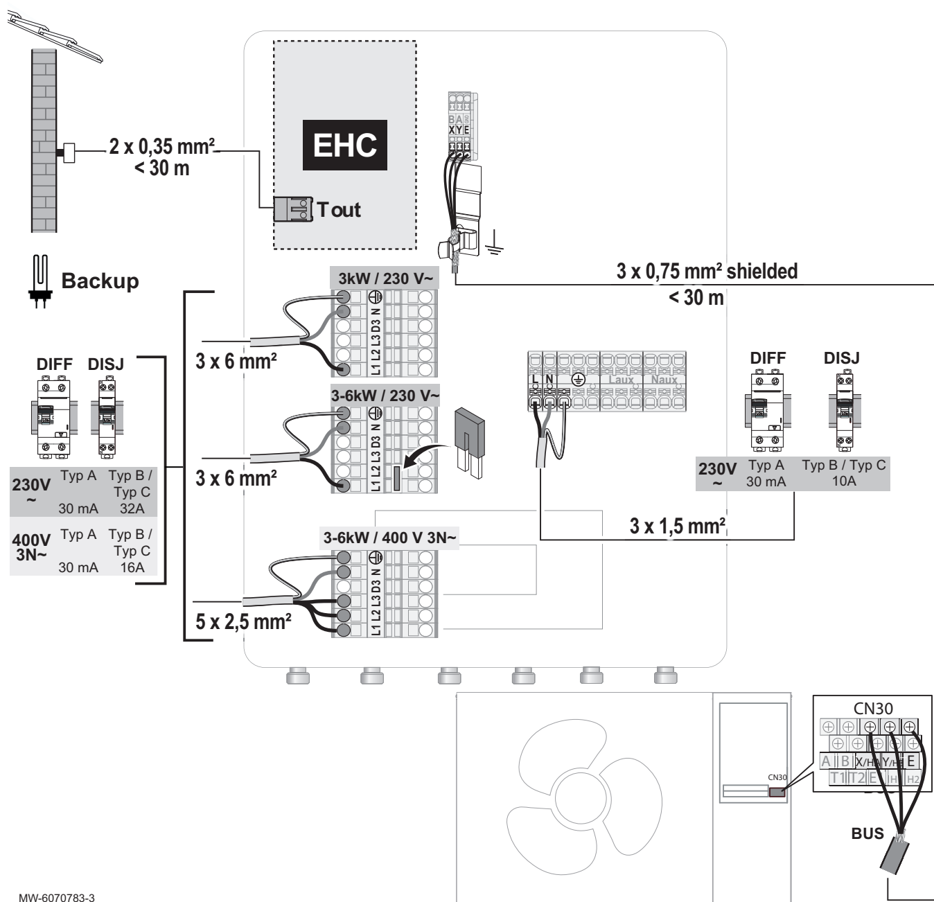
Fig.40 MONO AWHP3R et MIV-M /E avec résistance électrique 3-6 kW
