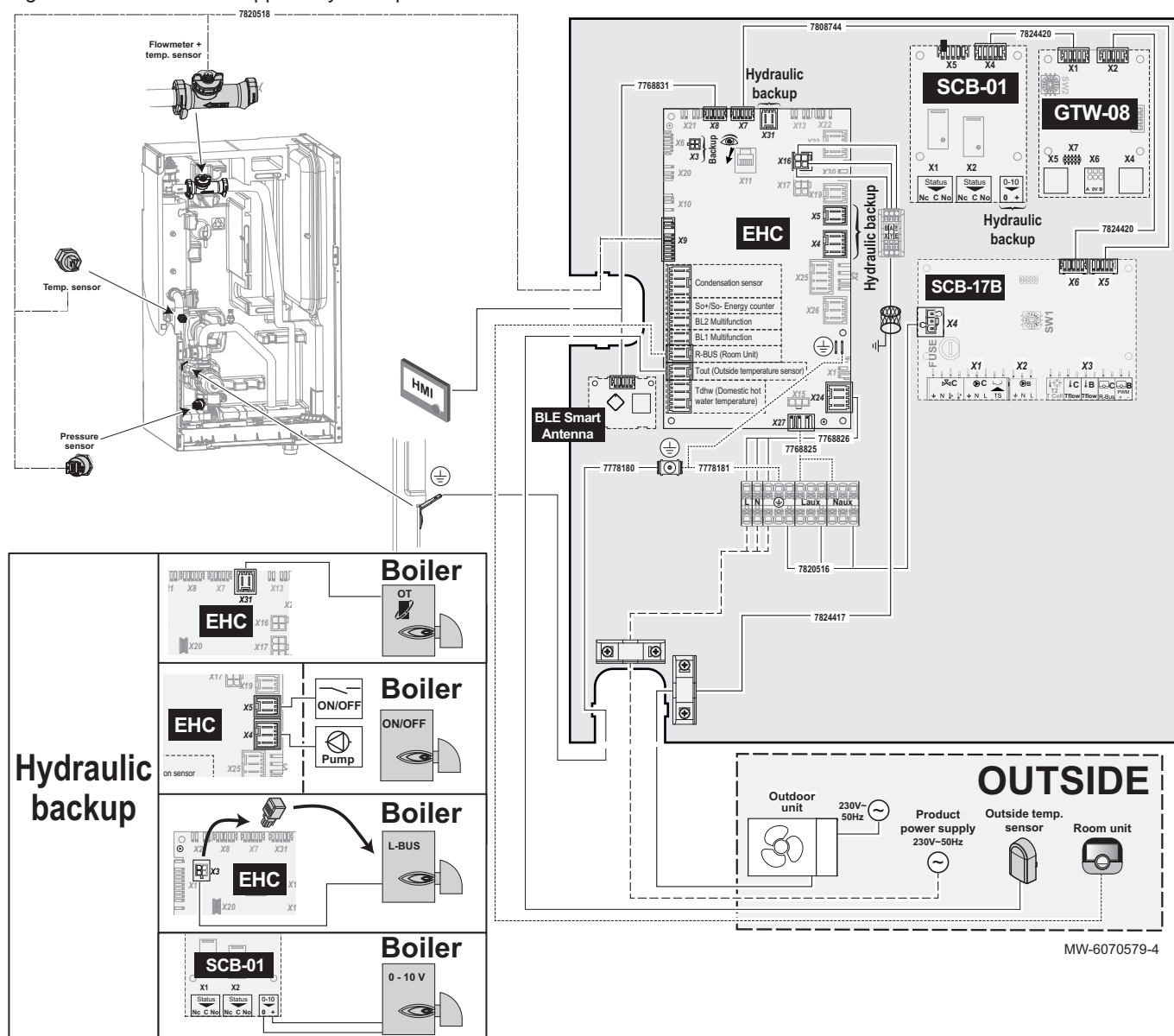
Fig.9 MIV-M /H avec appoint hydraulique
