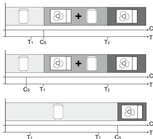
Fig.71 Influence des températures extérieures et de bivalence.
