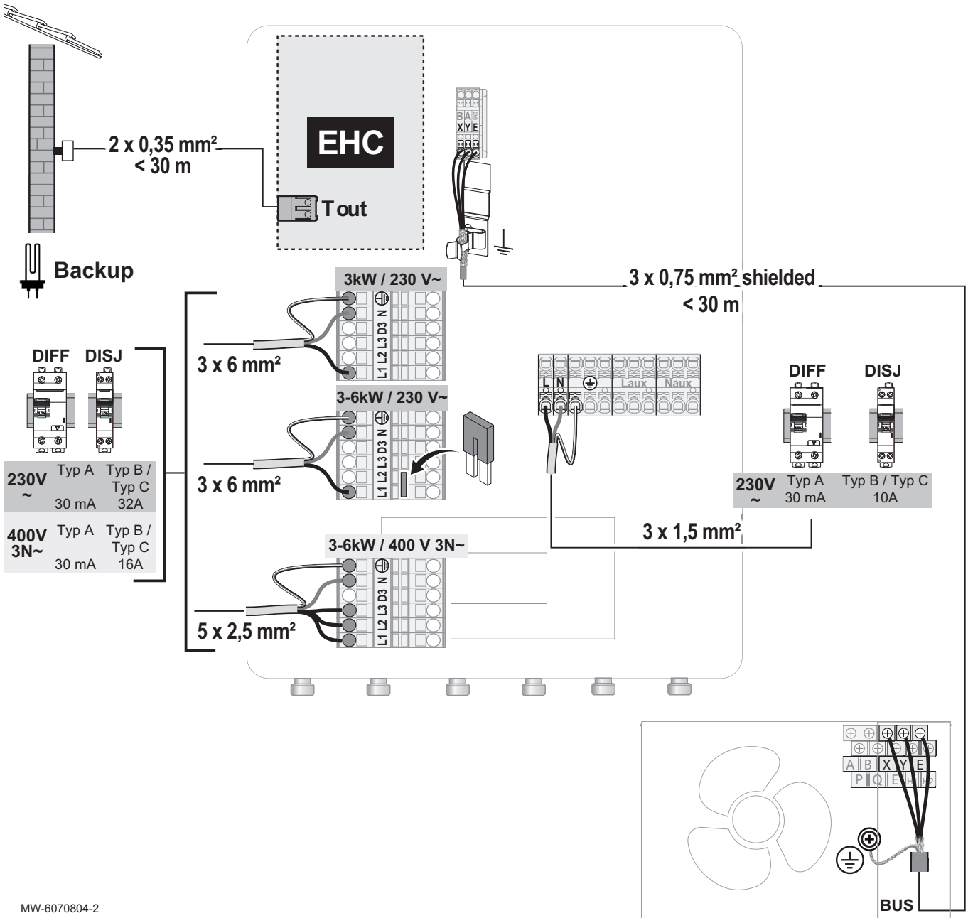
Fig.41 MONO AWHP2R et MIV-M /E avec résistance électrique 3-6 kW
