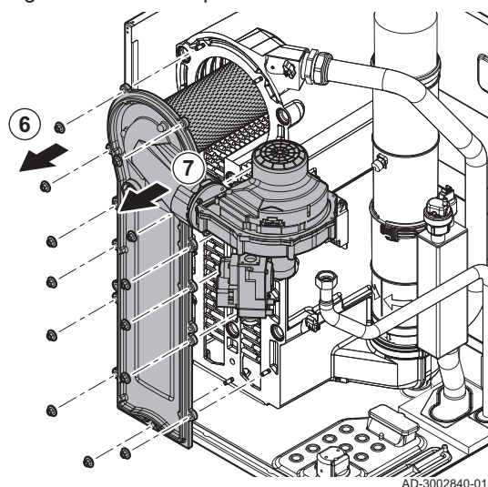
Fig.104 Retrait du panneau avant
