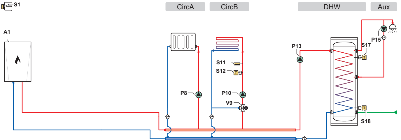
Fig.81 Schéma et composants - 6000254
