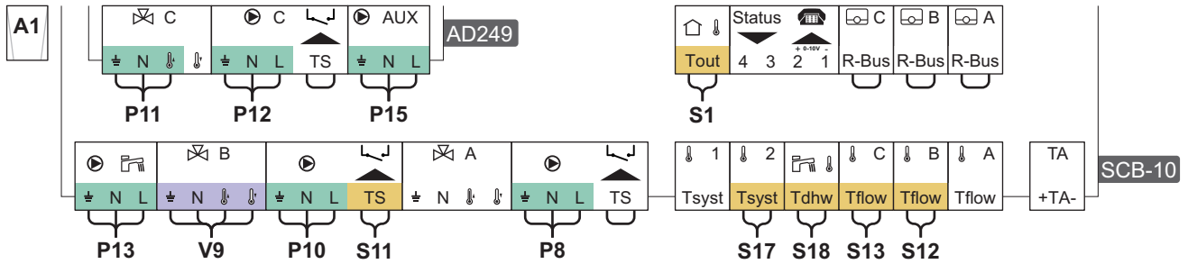
Fig.84 Raccordements électriques - Chaudière A1
