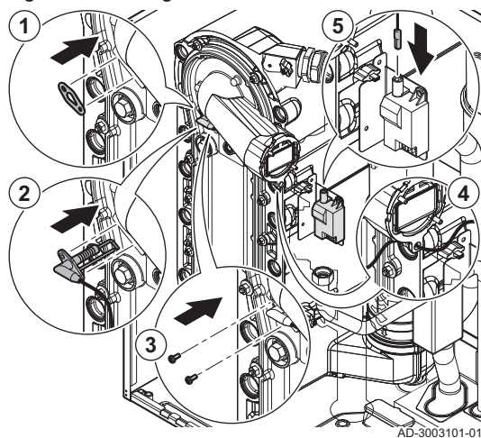
Fig.124 Montage de l'électrode
