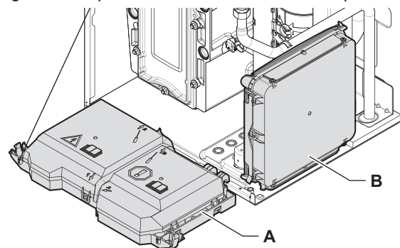
Fig.33 Emplacements des cartes électroniques
