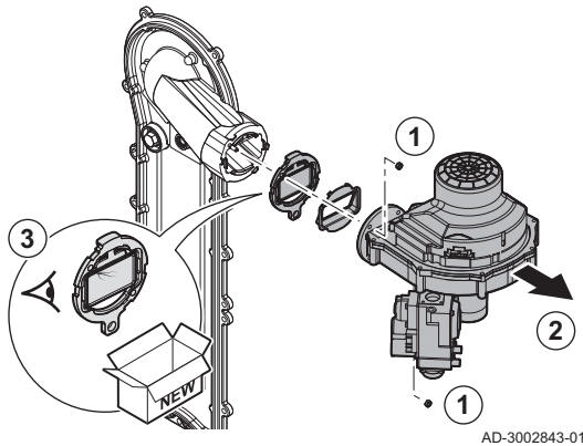
Fig.108 Contrôle du clapet antiretour
