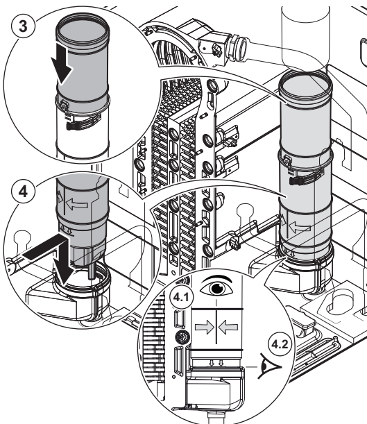
Fig.115 Mise en place du conduit de fumées
