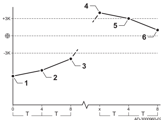
Fig.27 Commande traditionnelle d'une cascade
