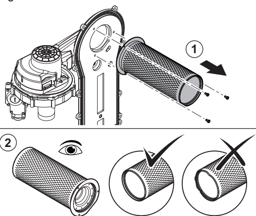
Fig.105 Contrôle du brûleur
