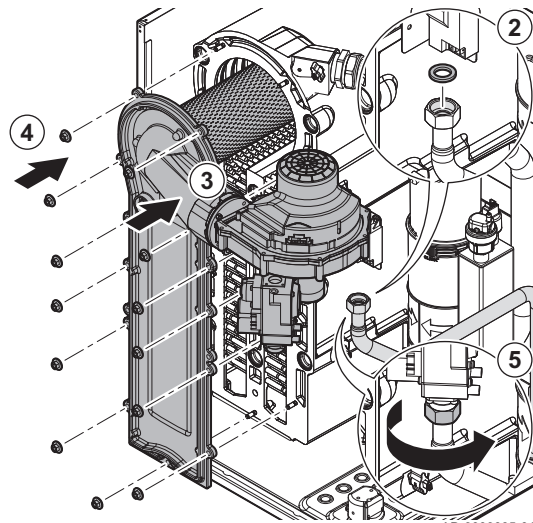
Fig.121 Montage de la plaque avant
