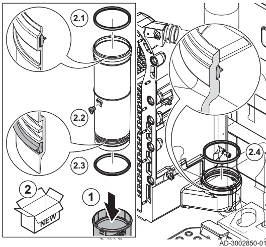
Fig.115 Mise en place du conduit de fumées
