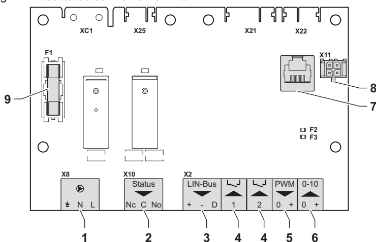
Fig.41 Carte de connexion CB-23
