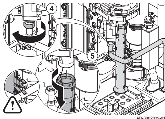
Fig.103 Démontage du bloc ventilateur
