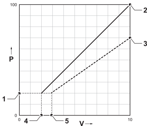
Fig.25 Graphique de régulation de la puissance
