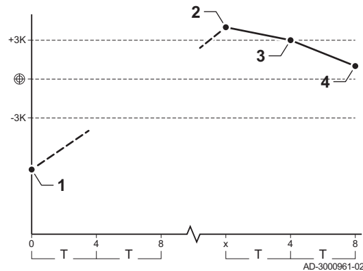
Fig.28 Commande d'une cascade en parallèle
