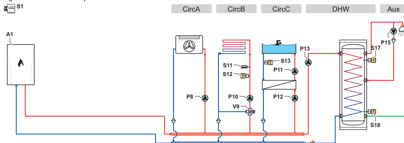
Fig.83 Schéma et composants - 6000255
