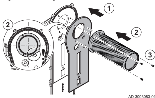
Fig.119 Montage du brûleur
