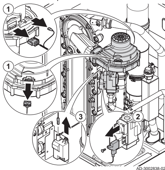
Fig.103 Démontage du bloc ventilateur
