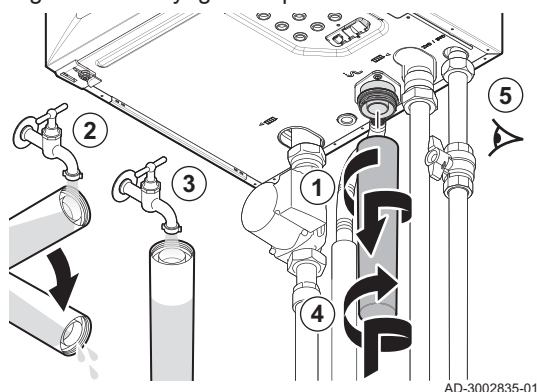
Fig.100 Nettoyage du siphon
