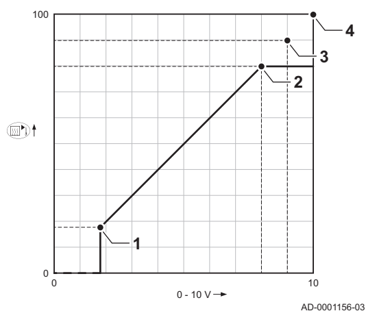
Fig.24 Graphique de régulation de la température
