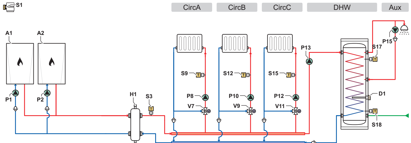
Fig.85 Schéma et composants - 6000256
