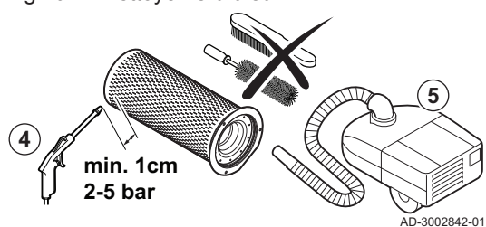
Fig.107 Nettoyer le brûleur
