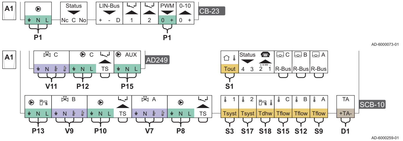
Fig.87 Raccordements électriques - Chaudière suiveuse A2
