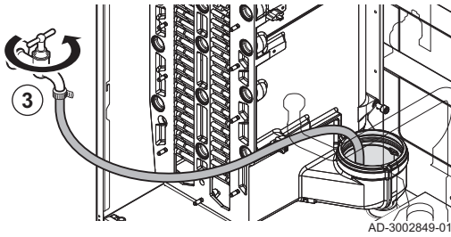
Fig.113 Rinçage du récupérateur de condensats
