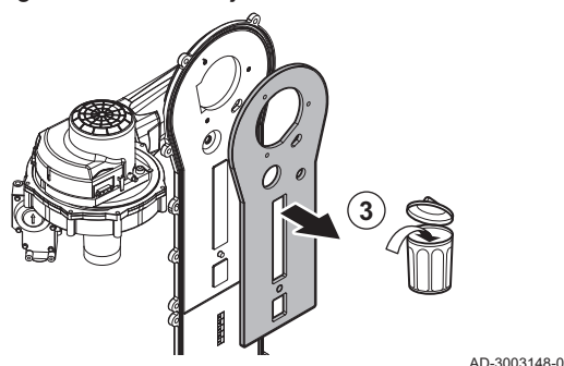
Fig.107 Nettoyer le brûleur
