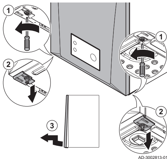
Fig.99 Dépose du panneau
