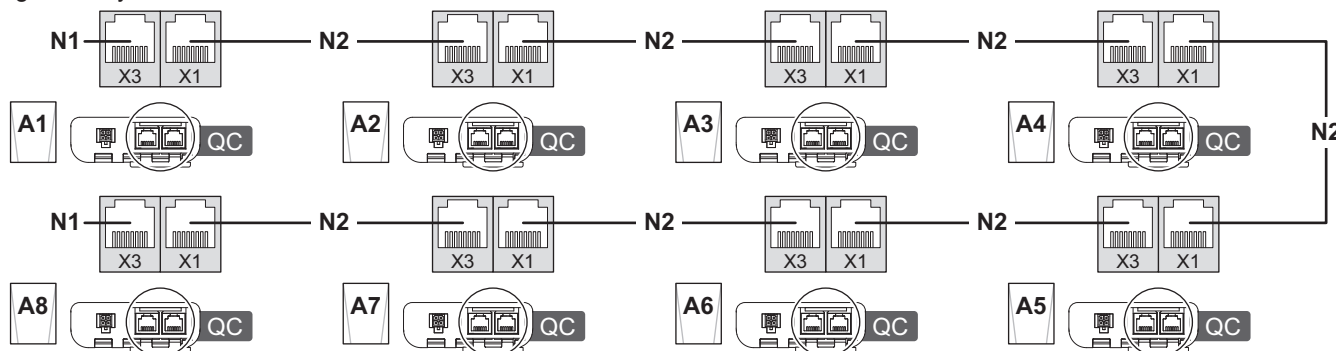
Fig.32 Système en cascade
