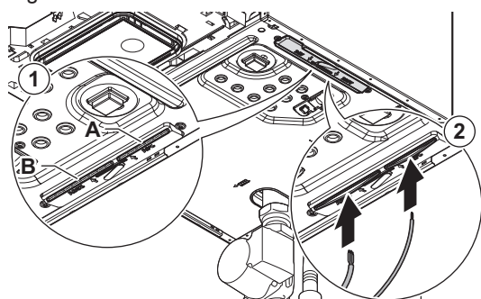
Fig.39 Cheminement des câbles
