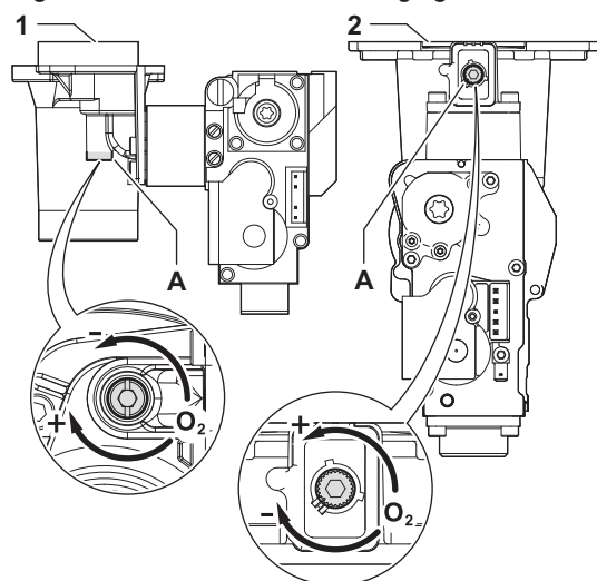
Fig.96 Position de la vis de réglage A
