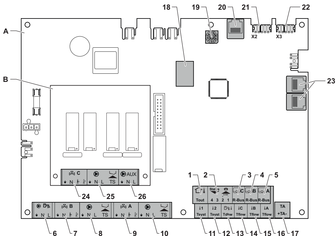
Fig.61 SCB-10 avec AD249
