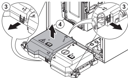
Fig.35 Soulever le couvercle
