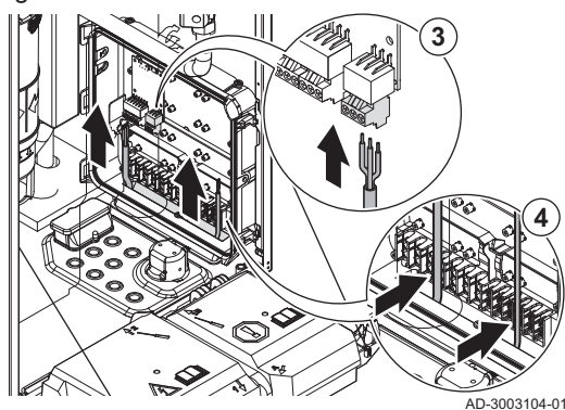
Fig.40 Connexion du câble
