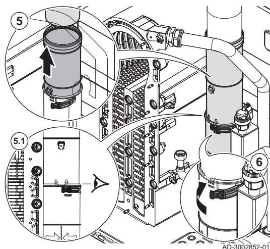
Fig.117 Réassemblage du conduit de fumées
