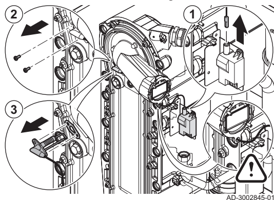
Fig.101 Remplacement de l'électrode d'ionisation/d'allumage
