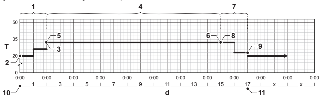
Fig.17 Courbe de séchage de la chape
