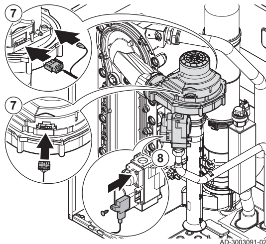
Fig.123 Raccordements électriques
