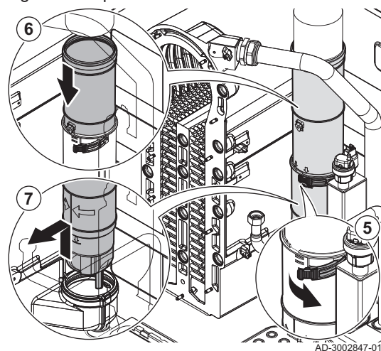
Fig.111 Dépose du conduit de fumées
