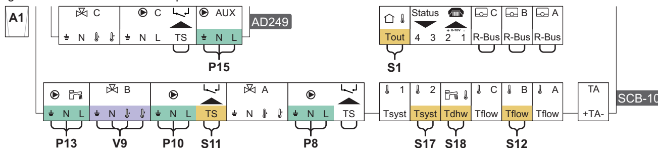
Fig.82 Raccordements électriques - Chaudière A1
