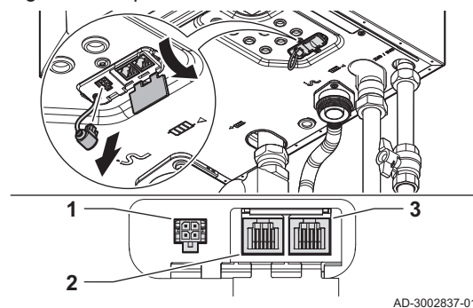
Fig.29 Emplacement du Quick connect
