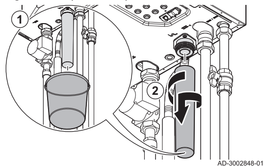
Fig.112 Dépose du siphon
