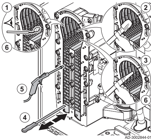
Fig.109 Nettoyage de l'échangeur de chaleur
