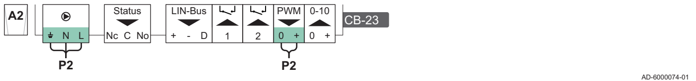
Fig.88 Connexions S-Bus - Chaudière pilote A1 à Chaudière suiveuse A2
