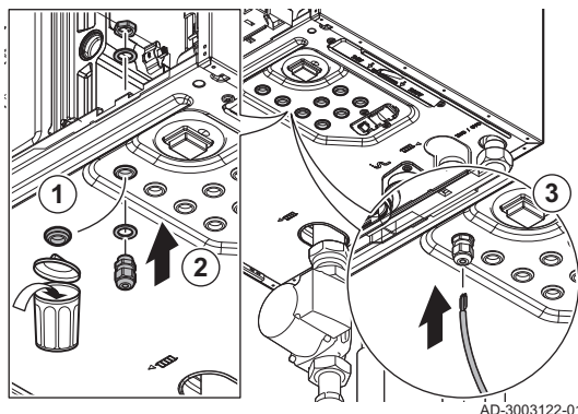
Fig.36 Cheminement des câbles
