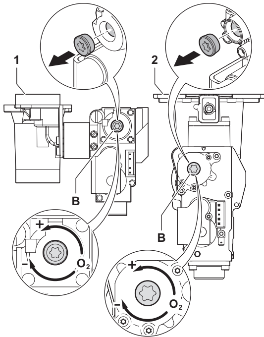
Fig.98 Position de la vis de réglage B
