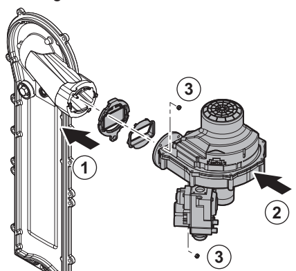
Fig.118 Montage du ventilateur et du bloc vanne gaz
