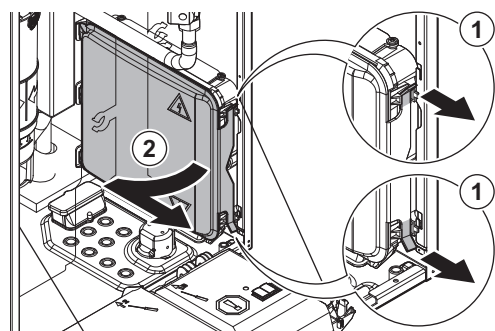
Fig.38 Accès au boîtier pour cartes d'extension
