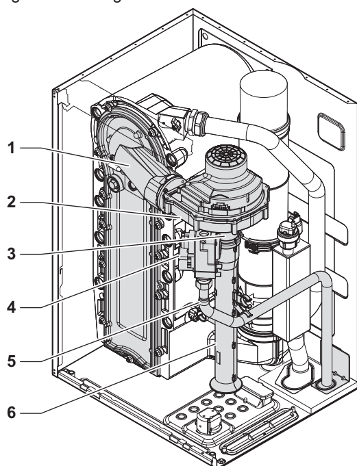
Fig.3 Unité gaz-air
