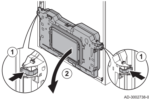
Fig.115 Basculer le boîtier de commande vers l'avant
