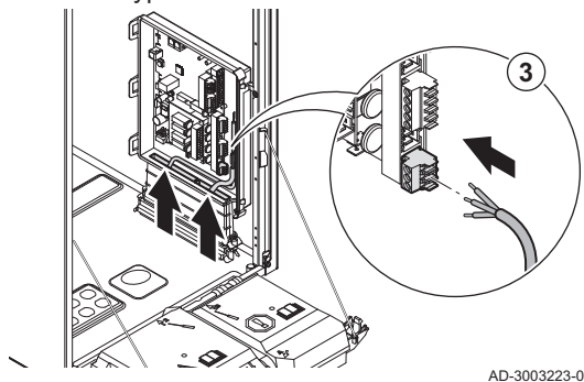
Fig.60 Cheminement des câbles à l'intérieur du boîtier pour cartes d'extension pour les chaudières de type 35 - 50 - 60 - 70
