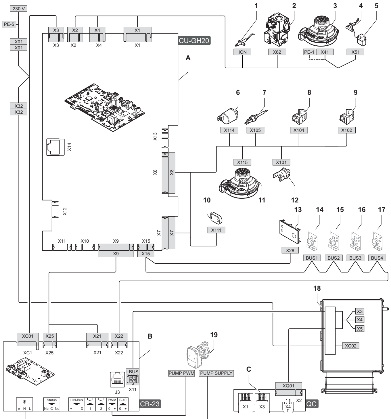
Fig.130 Schéma électrique pour les chaudières de type 35 - 50 - 60 - 70
