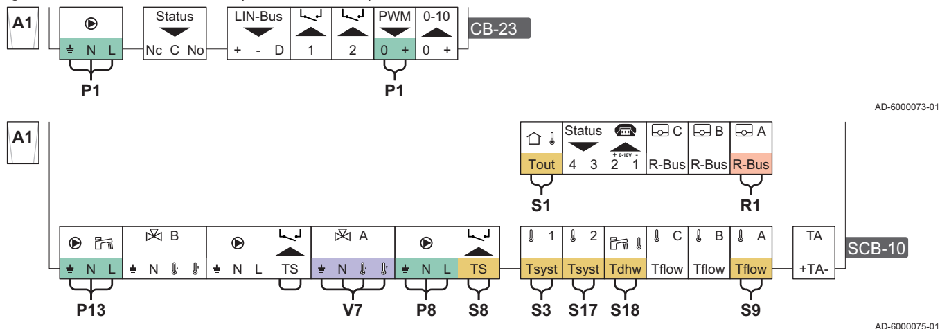
Fig.29 Raccordements électriques - Chaudière pilote A1
