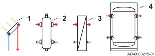
Fig.24 Séparateur hydraulique
