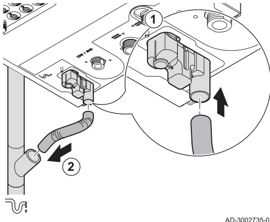
Fig.43 Raccordement du tube d'évacuation des condensats
