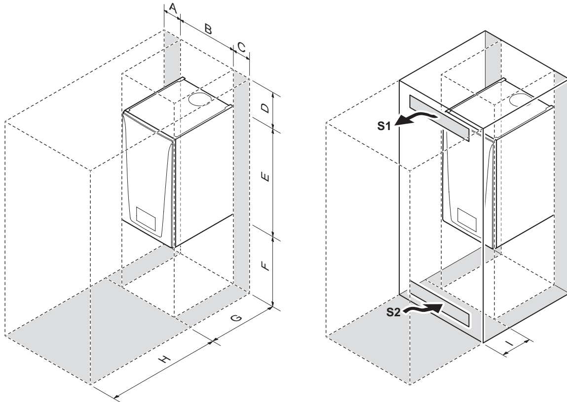
Fig.7 Exigences relatives à l'emplacement
