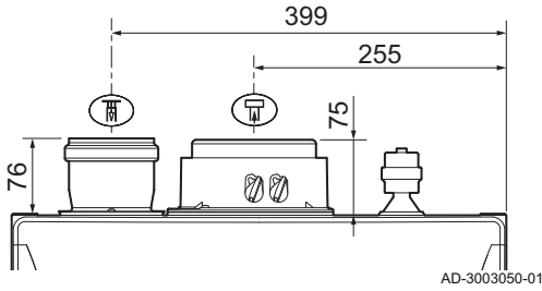
Fig.47 Dimensions du kit de séparation des fumées
