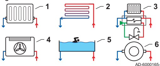
Fig.22 Consommateurs
