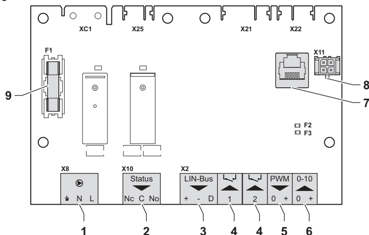
Fig.61 Carte de connexion CB-23
