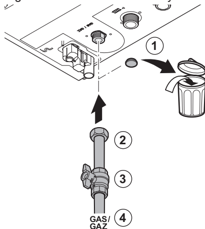
Fig.45 Raccordement du tuyau de gaz
