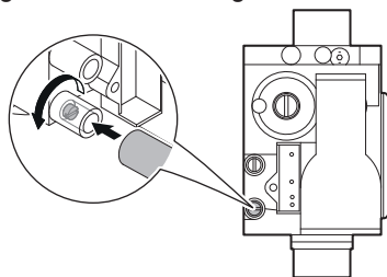
Fig.94 Bloc vanne gaz 35 - 50 - 60 - 70
