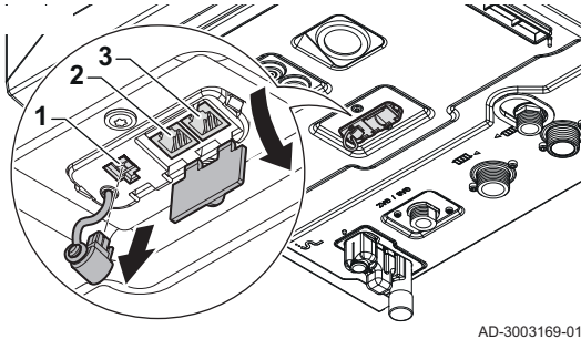
Fig.48 L'emplacement du Quick connect
