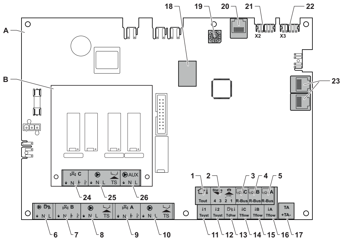
Fig.81 SCB-10 avec AD249
