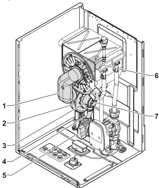
Fig.3 Gaz-air
