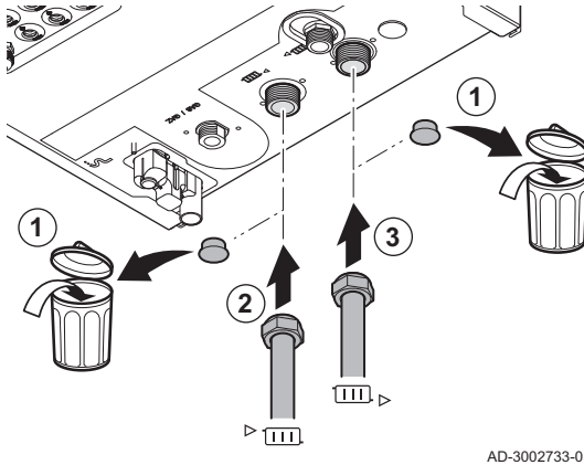
Fig.42 Raccordement du départ et du retour du chauffage central
