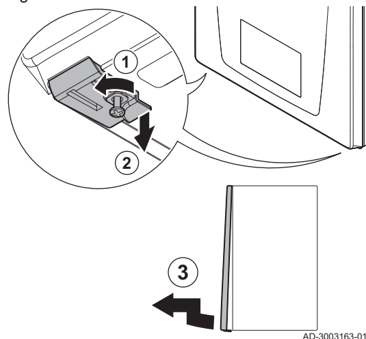
Fig.114 Ouvrir la chaudière
