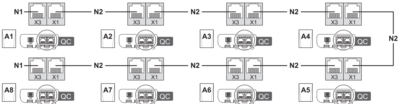
Fig.51 Système en cascade
