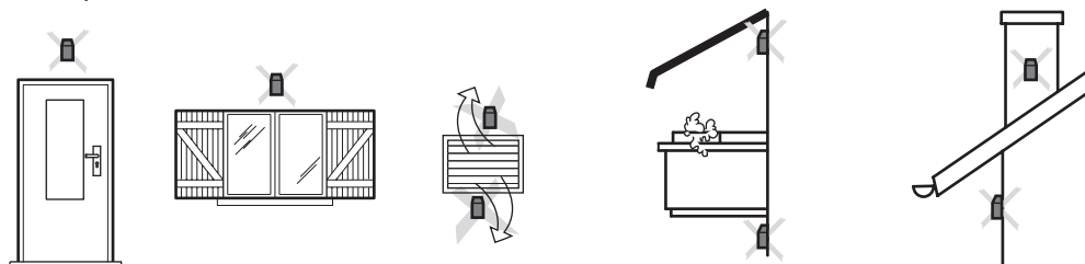
Fig.40 Emplacements déconseillés
