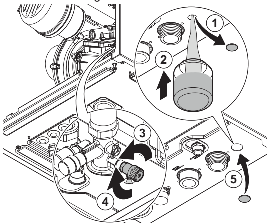
Fig.116 Ouvrir le robinet de vidange de l'échangeur de chaleur
