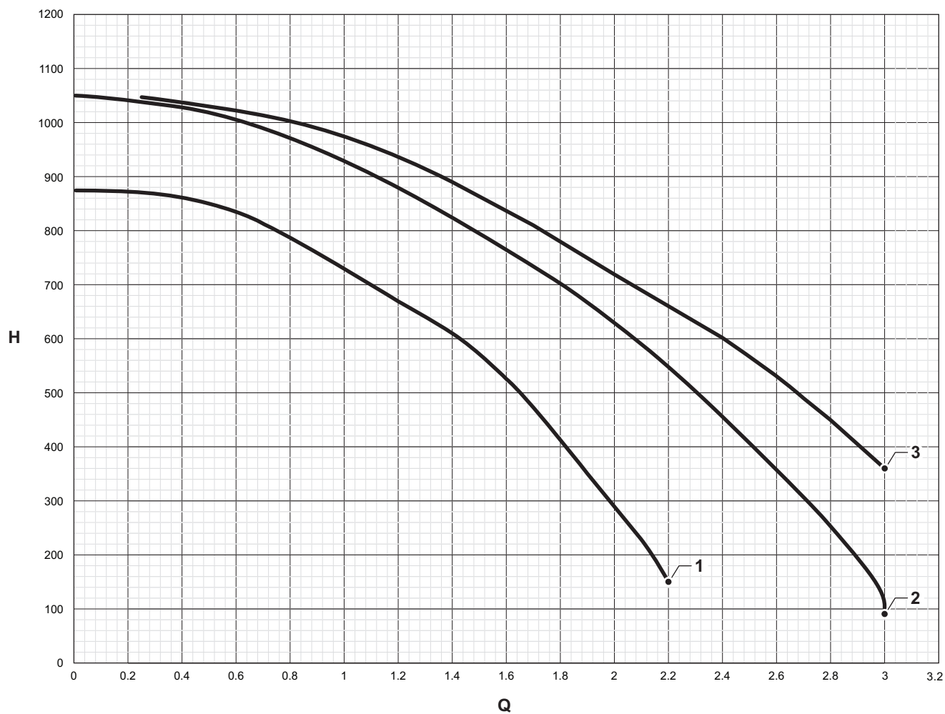
Fig.131 Pression disponible
