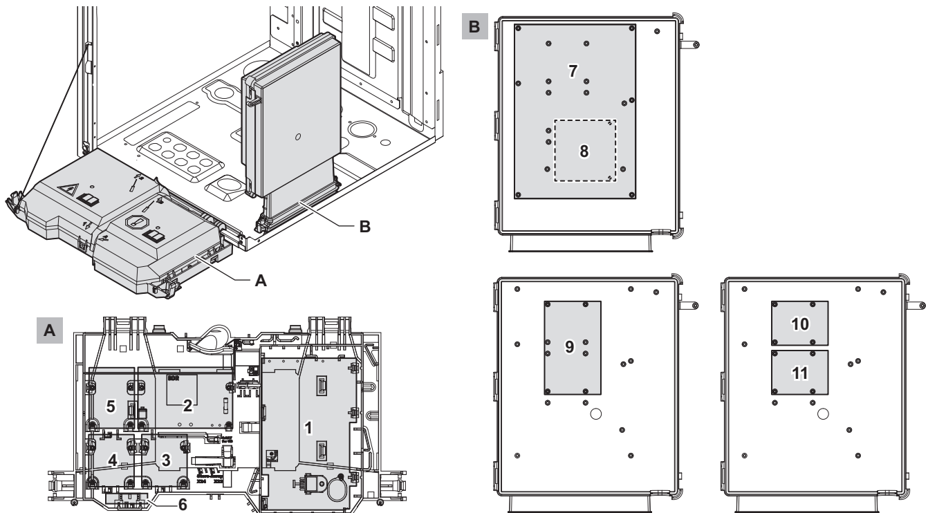
Fig.57 Emplacements des cartes électroniques dans les chaudières de type 35 - 50 - 60 - 70.
