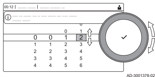
Fig.108 Niveau installateur
