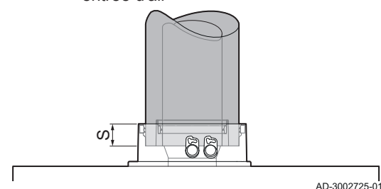
Fig.46 Raccordement du tuyau de fumée/entrée d'air
