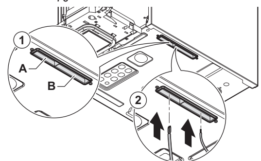
Fig.59 Cheminement des câbles vers le boîtier pour cartes d'extension pour les chaudières de type 35 - 50 - 60 - 70
