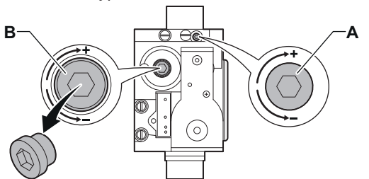
Fig.102 Bloc vanne gaz dans les chaudières de type : 35 - 50 - 60 - 70
