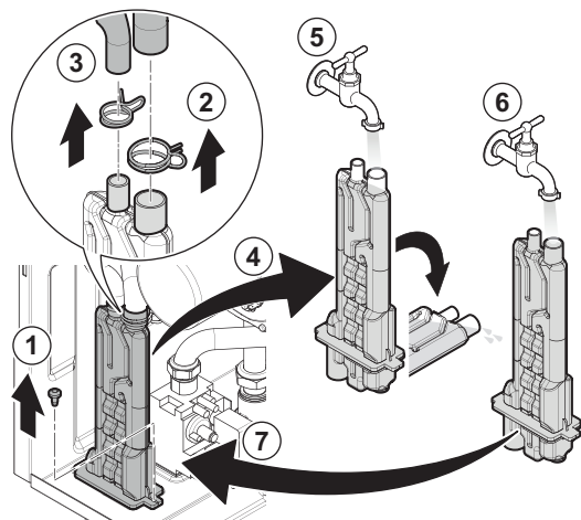
Fig.117 Nettoyer le siphon.
