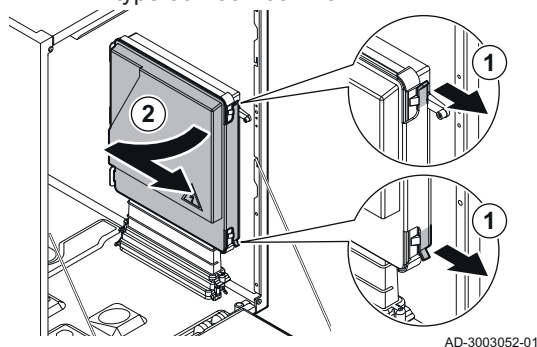
Fig.58 Accès au boîtier pour cartes d'extension dans les chaudières de type 35 - 50 - 60 - 70.
