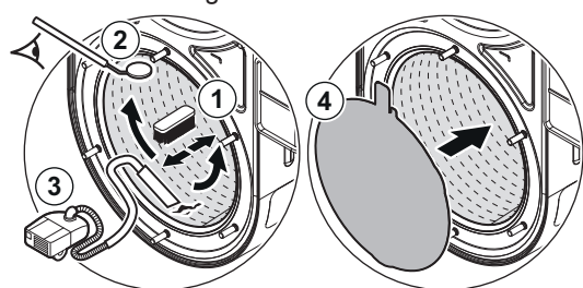
Fig.53 Brossage et aspiration de l'échangeur de chaleur
