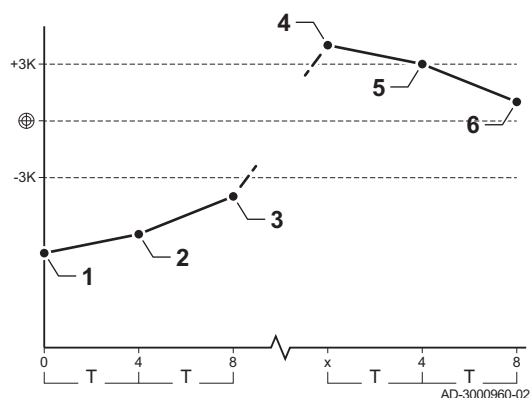
Fig.28 Mode de fonctionnement en cascade traditionnelle
