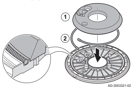
Fig.55 Installation de l'isolation du brûleur et du joint du cordon en fibre de verre.
