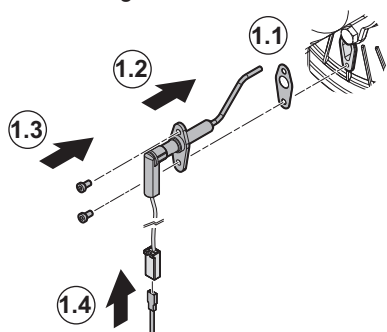
Fig.60 Fixation de l'électrode d'ionisation et d'allumage
