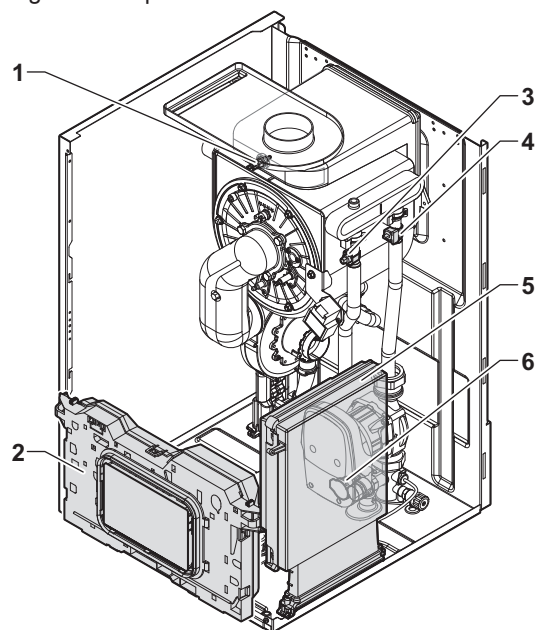
Fig.4 Capteurs et boîtiers
