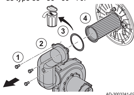
Fig.51 Retrait du brûleur des chaudières de type 35 - 50 - 60 - 70.
