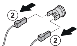
Fig.42 Retrait du câble de l'électrode d'ionisation
