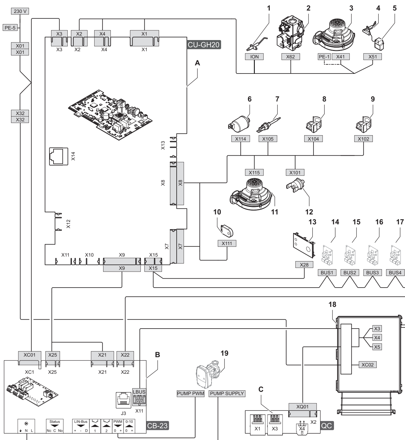
Fig.65 Schéma électrique pour les chaudières de type 35 - 50 - 60 - 70
