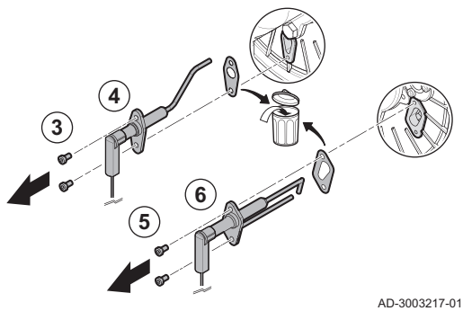
Fig.48 Retrait des électrodes
