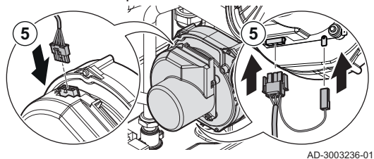
Fig.59 Installation des branchements électriques du ventilateur
