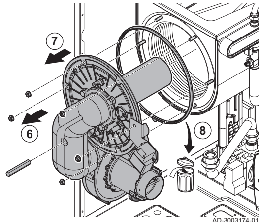
Fig.45 Retrait de la plaque avant
