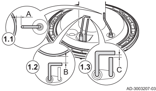
Fig.46 Contrôle des distances des électrodes
