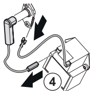
Fig.43 Retrait du câble d'allumage
