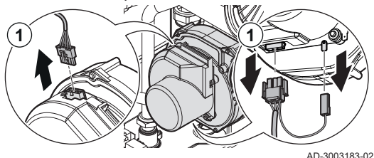
Fig.41 Retrait des branchements du thermostat de sécurité
