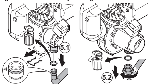
Fig.44 Retrait du tuyau de gaz du venturi
