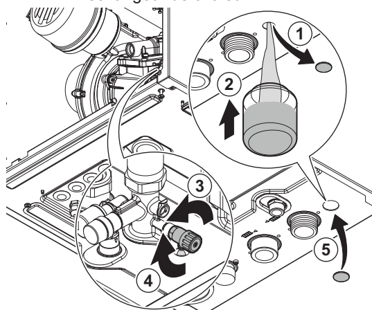
Fig.38 Ouvrir le robinet de vidange de l'échangeur de chaleur
