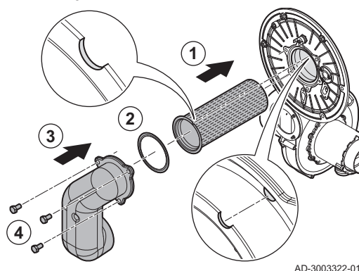
Fig.56 Montage du brûleur pour les chaudières de type 35 - 50 - 60 - 70.
