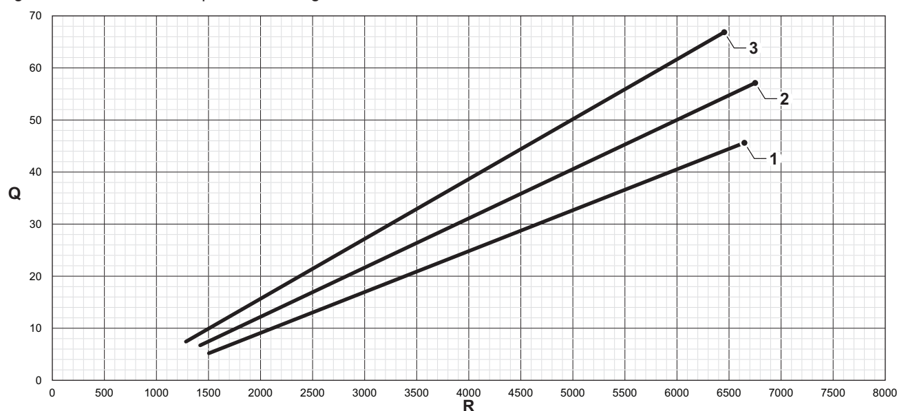
Fig.24 Entrée maximale pour le chauffage central
