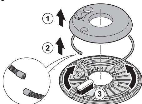
Fig.52 Retrait de l'isolation du brûleur
