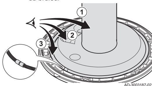
Fig.50 Contrôle du brûleur et de l'isolation du brûleur
