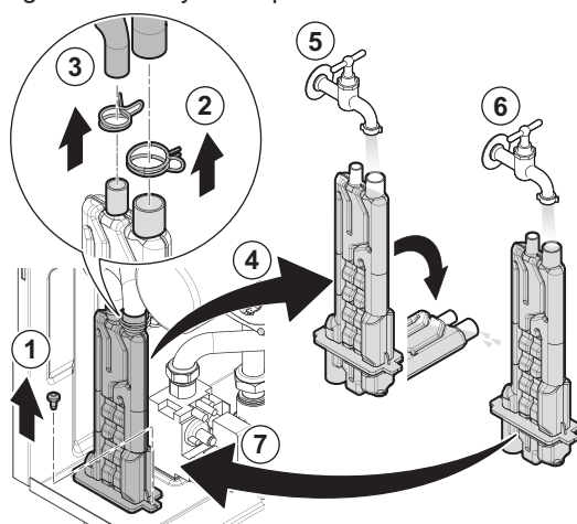
Fig.39 Nettoyer le siphon.
