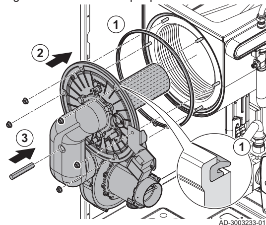
Fig.57 Fixation de la plaque avant
