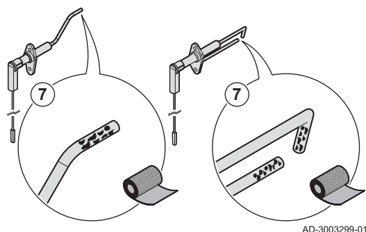
Fig.49 Nettoyage des électrodes
