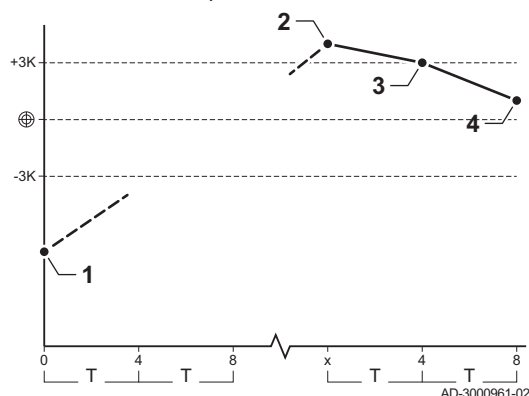
Fig.29 Mode de fonctionnement en cascade parallèle
