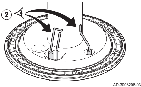
Fig.48 Retrait des électrodes
