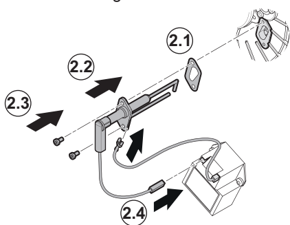
Fig.61 Fixation de l'électrode d'ionisation et d'allumage
