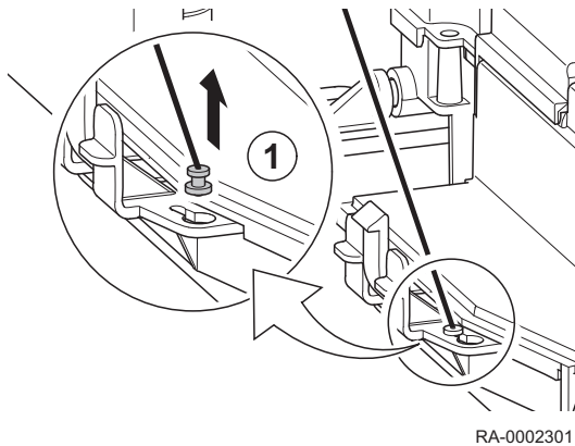
Fig.54 Ouverture du boîtier de commande
