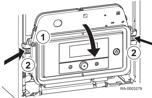
Fig.52 Déverrouillage du boîtier de commande
