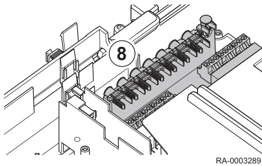
Fig.25 Carte de connexion CB
