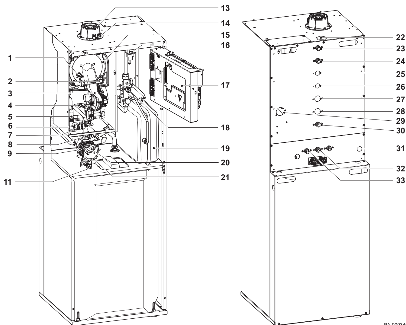
Fig.5 Vues de chaudière
