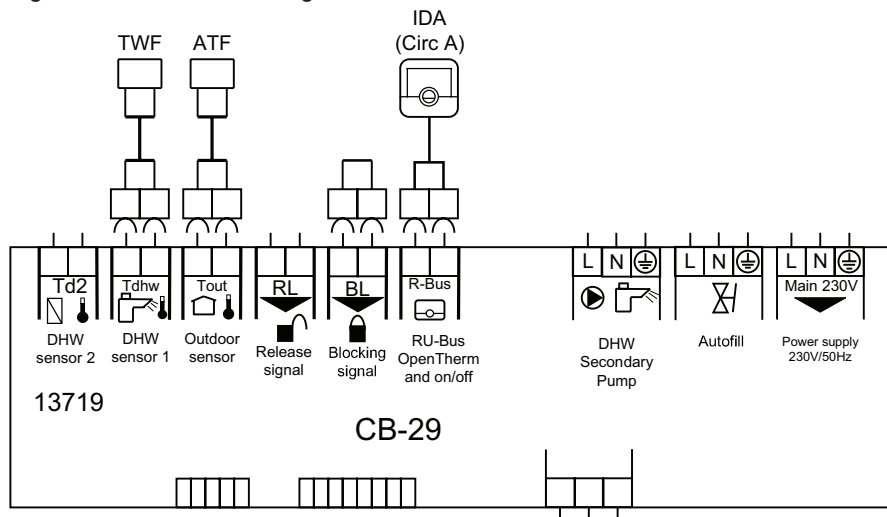
Fig.15 Schéma de câblage
