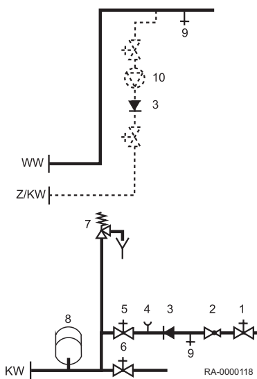
Fig.17 Raccord d'eau froide
