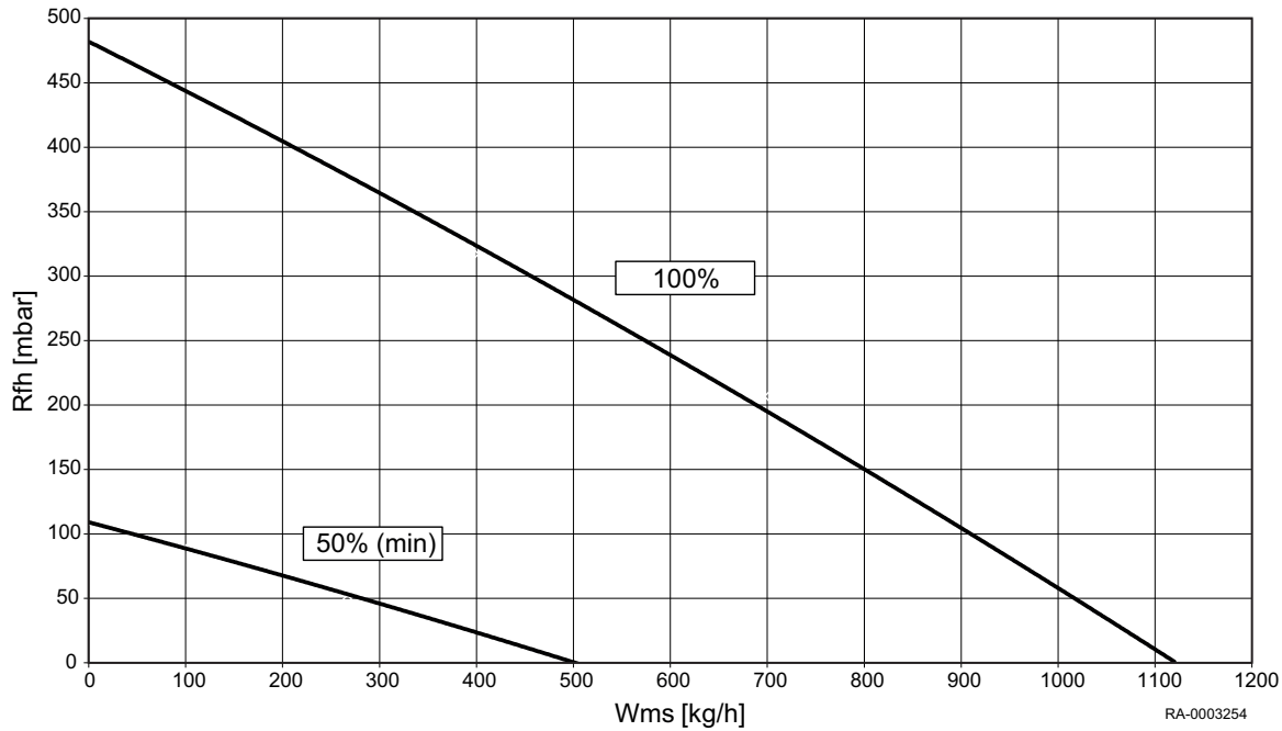
Fig.1 Pression d'alimentation résiduelle EGC EVO 25 B
