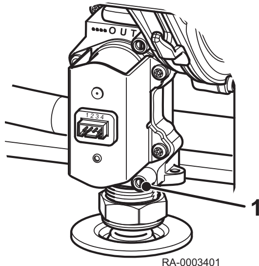
Fig.31 Bloc gaz EGC EVO
