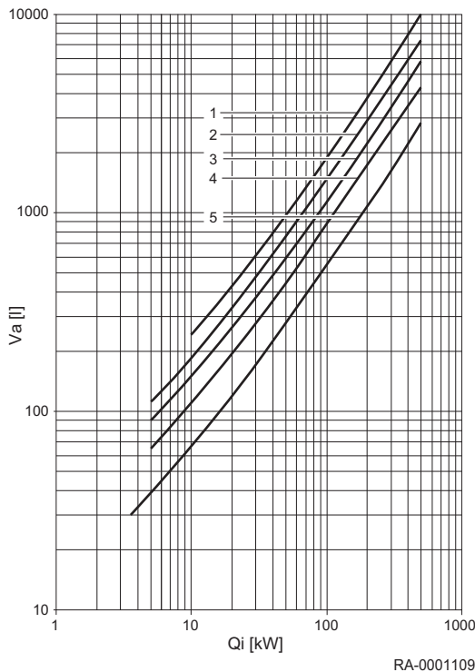
Fig.13 Détermination du volume de l'installation
