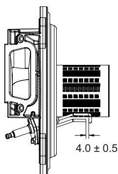
Fig.56 Distance des électrodes
