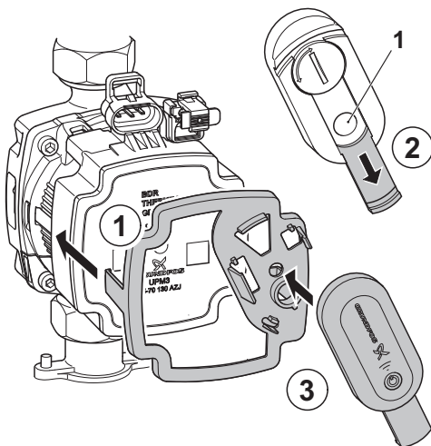
Fig.32 Installation de l'ALPHA Reader
