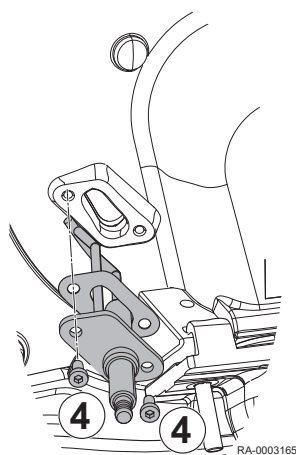
Fig.58 Retrait de l'électrode d'allumage et d'ionisation
