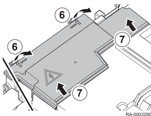
Fig.24 Déposer le capot supérieur du boîtier
