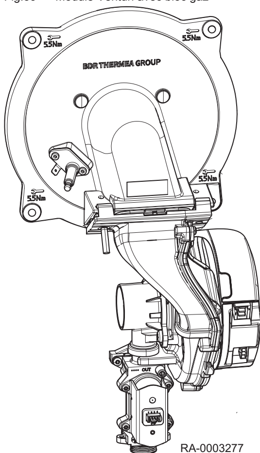
Fig.59 Module Venturi avec bloc gaz
