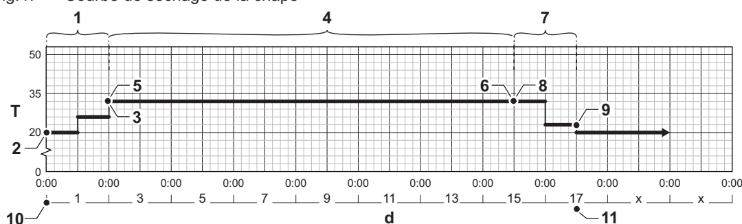
Fig.47 Courbe de séchage de la chape
