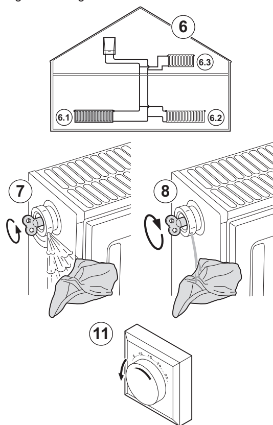
Fig.57 Purge de l'installation
