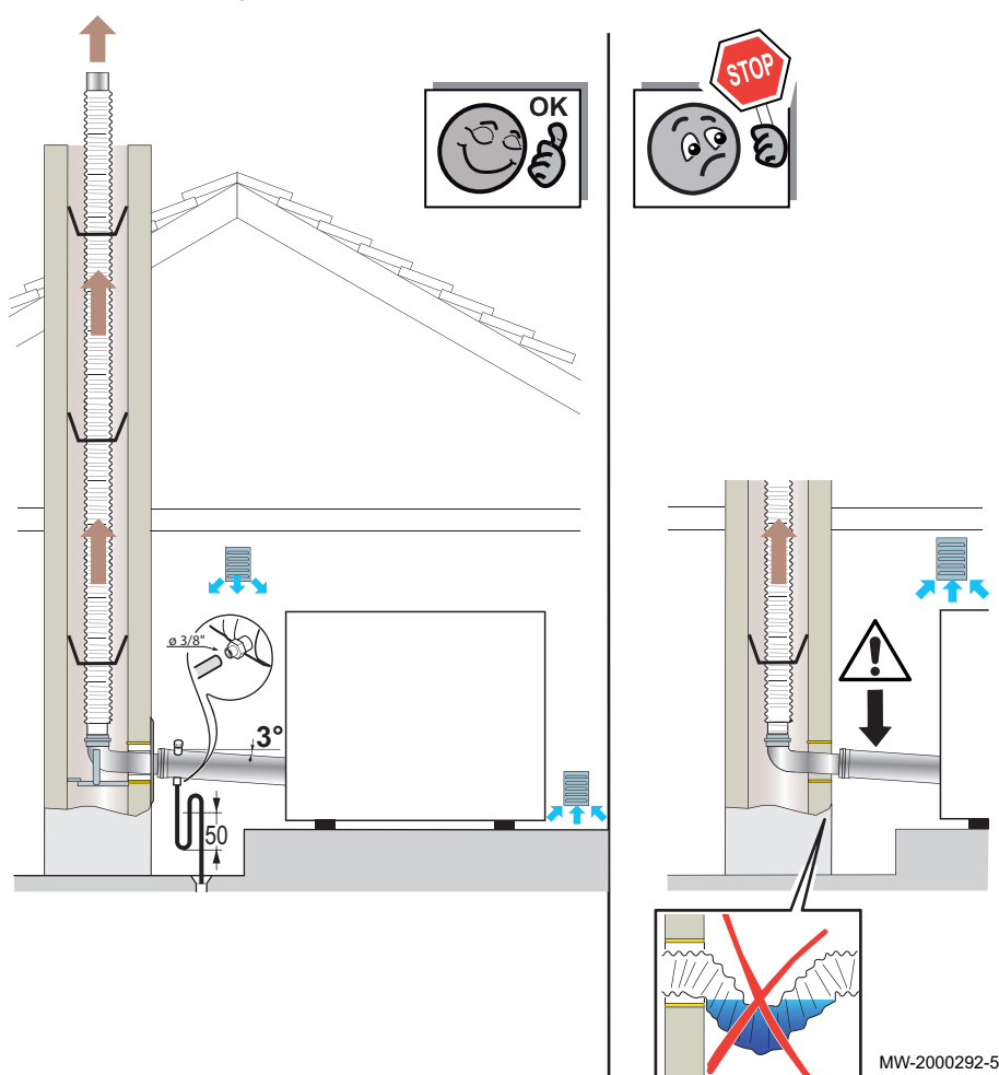
Fig.16 Raccordement de type B 23 en flexible - Conduits de fumées (air comburant pris dans la chaufferie)
