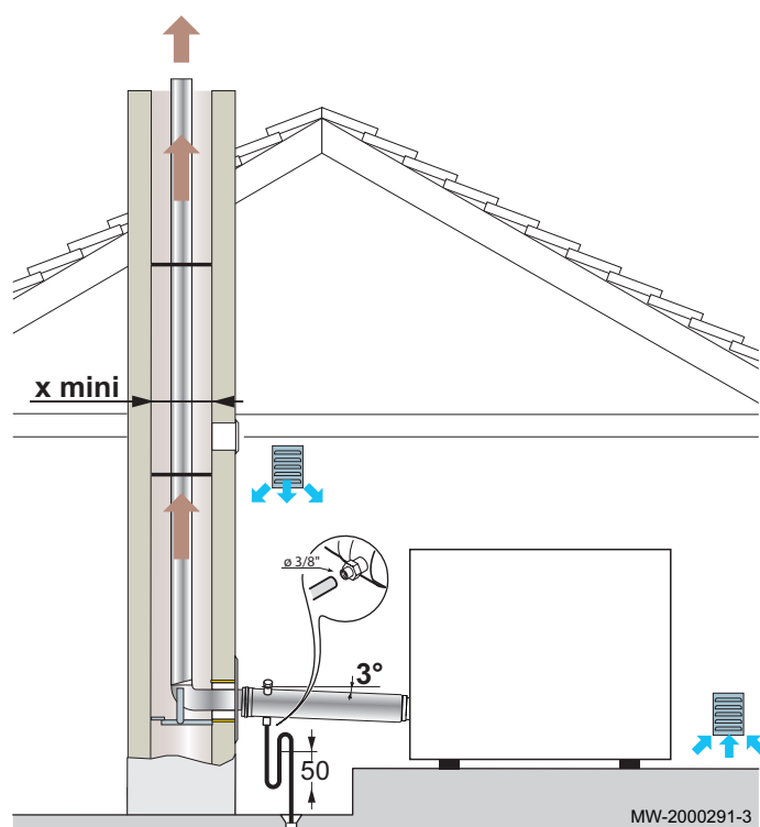
Fig.15 Raccordement de type B 23 en rigide - Conduits de fumées (air comburant pris dans la chaufferie)
